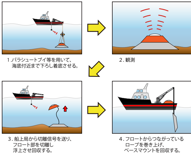
リカバリーポッド方式 - AL200/AL500 -
